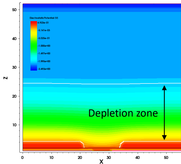
Bias: -2 V
