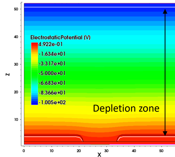
Bias: -100 V
