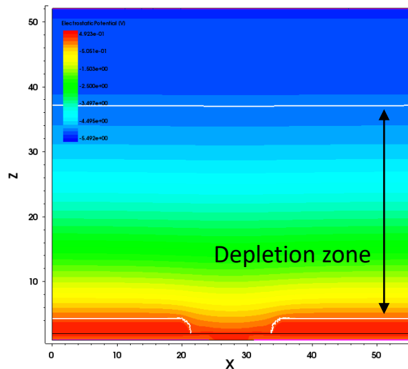
Bias: -5 V
